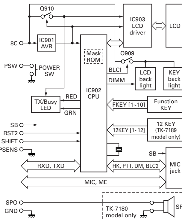
Fig. 7 Display circuit
